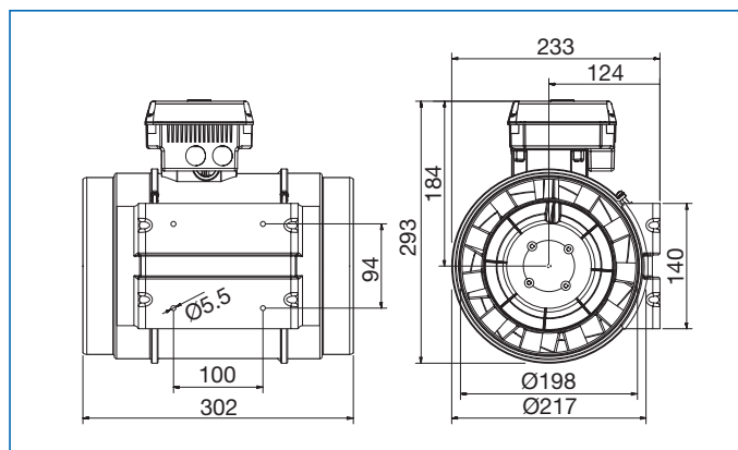
TD-800/200 ECOWATT
