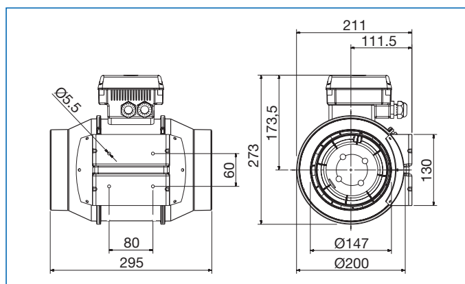
TD-500/150 ECOWATT
