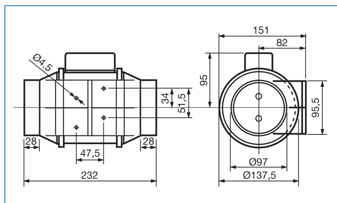
TD-160/100 ECOWATT
